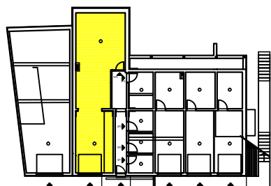
TLOCRT PODRUMA
