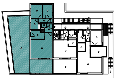
TLOCRT PRIZEMLJA
